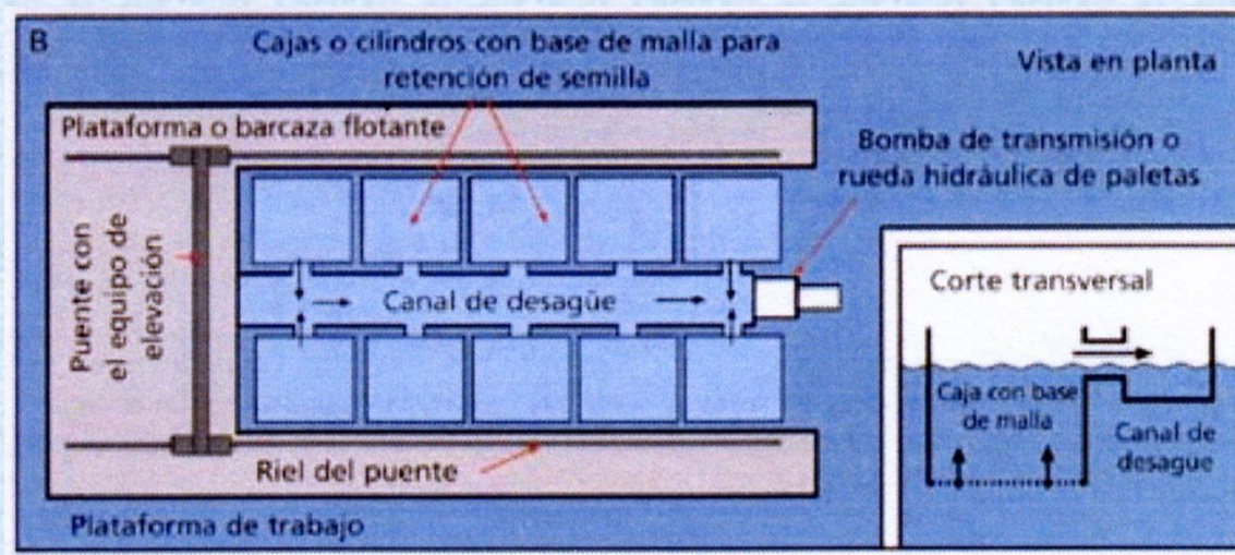
Esquema dun semilleiro sobre plataforma na zona marítima
