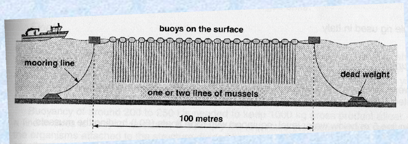
Esquema dunha líña de cultivo en superficie
