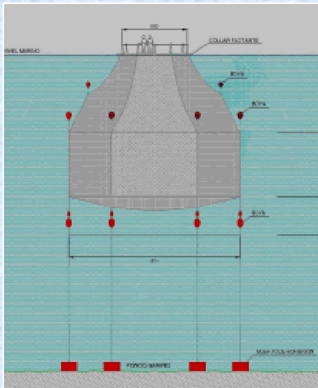
Gaiola sumerxible tipo Refa
